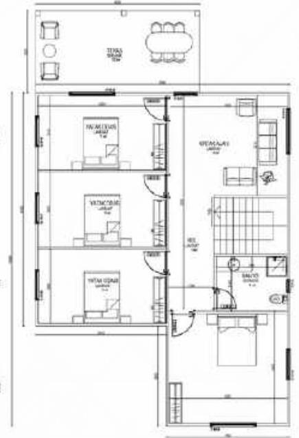
BİRİNCİ KAT ALANI: 129 M 2
